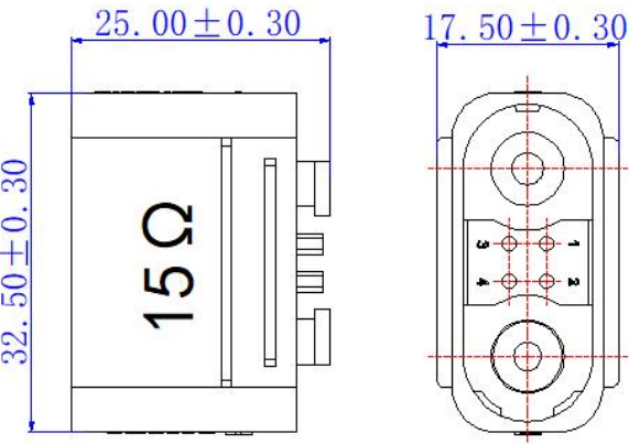
互配尺寸
