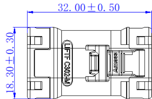
互配尺寸
