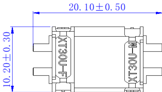
互配尺寸 Matching size
