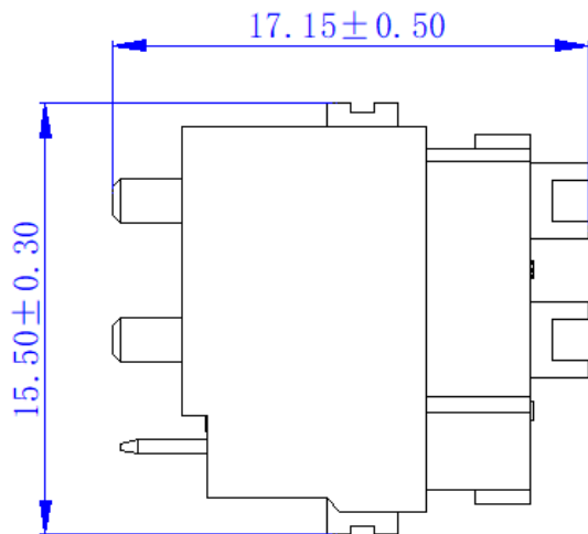
互配尺寸 Matching size
