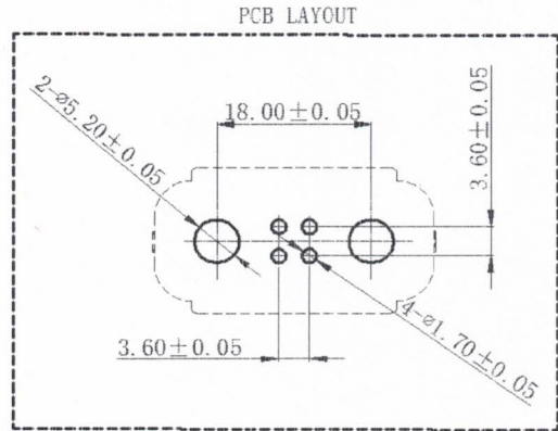
PCB 安装孔示意图
