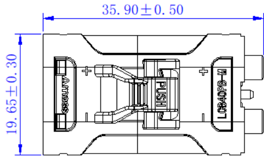
互配尺寸
