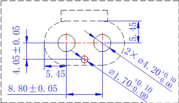
互配尺寸
