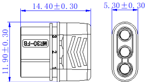
互配尺寸 Matching size
