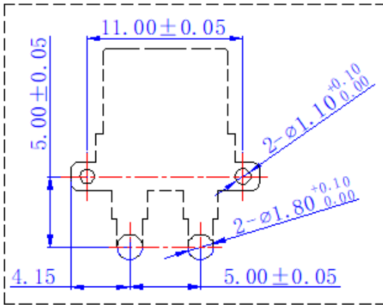
互配尺寸 Matching size
