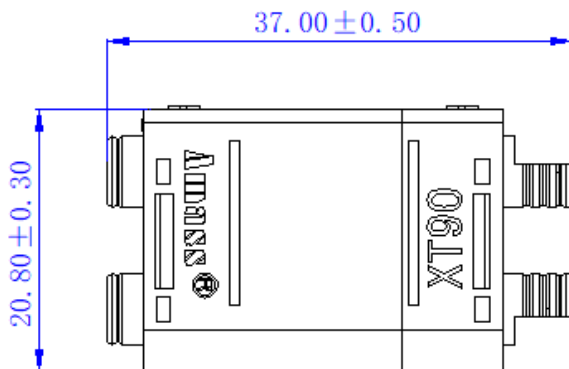
互配尺寸 Matching size
