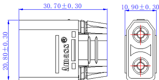
互配尺寸 Matching size
