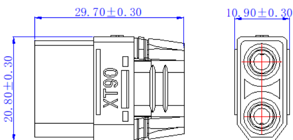
互配尺寸 Matching size
