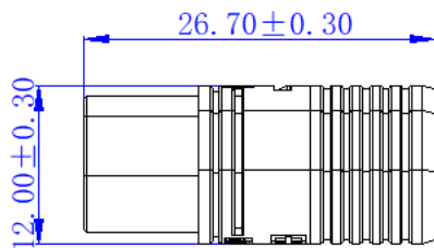
互配尺寸 Matching size
