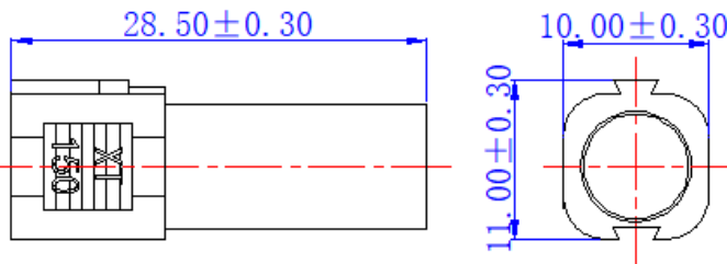
互配尺寸 Matching size
