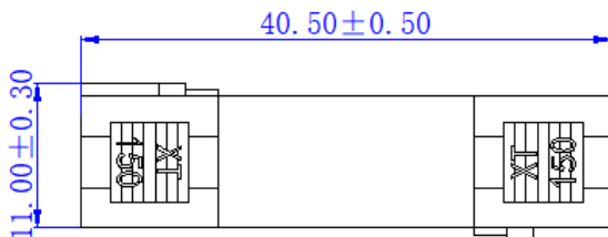
互配尺寸 Matching size
