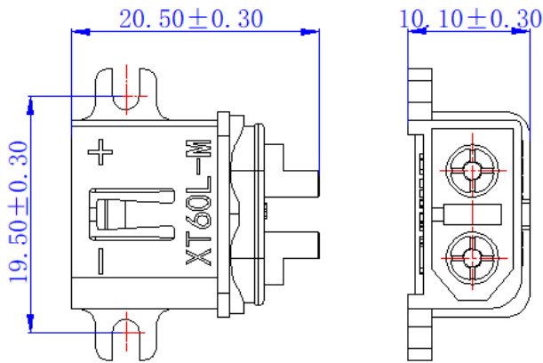
互配尺寸 Matching size
