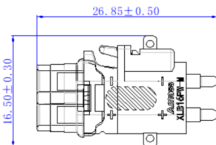
与 F 端带后盖互配尺寸 Matching size with back
