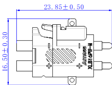
与 F 端带后盖互配尺寸 Matching size with back
