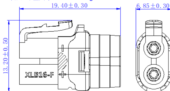
互配尺寸 Matching size
