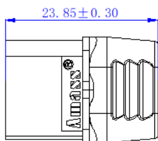
互配尺寸 Matching size
