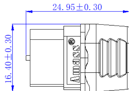
互配尺寸 Matching size
